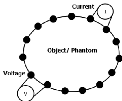
Figure 1. EIT Diagram
